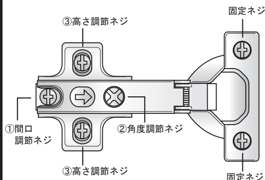
ヒンジ：上面図
